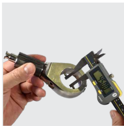
Medición interior con S_Cal EVO Smart PJ
