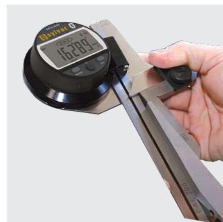
Medición con accesorio tipo 820-2461
