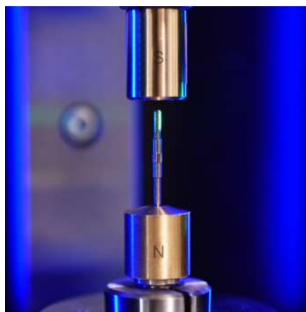
Medición de piezas pequeñas por levitación magnética en SCAN S25T
