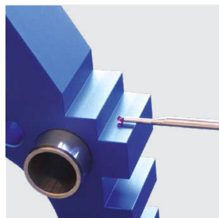
Medición de alturas y espesores con el palpador standard 930-2101
