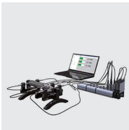
Conexión de palpador PC por MB-RS
